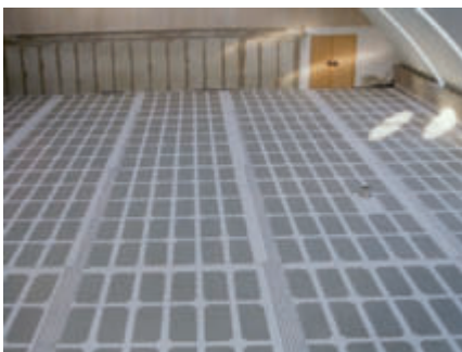
Modul Klimaböden sorgen auch bei Sportstätten, wie hier in einer Turnhalle, für Behaglichkeit der Marke Harreither.
